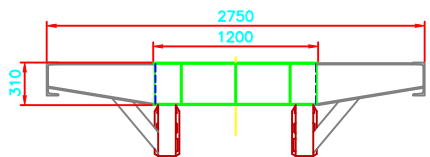
Doorsnede diepbed
