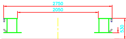
Doorsnede diepbed
